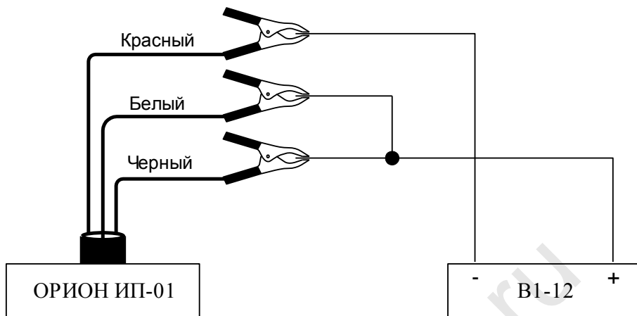
Рисунок 9.1 – Схема подключения к прибору В1-12
